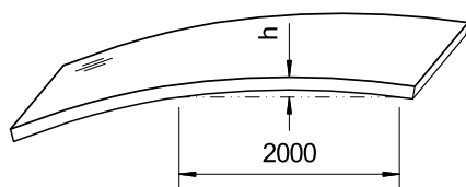
Abb. 118: Längskrümmung in Richtung der Dicke
