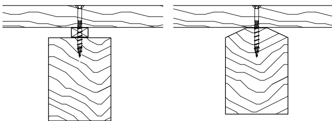
Abb. 106: Möglichkeiten um die Kontaktfläche zwischen Dielung und Unterkonstruktion zu reduzieren. Die Feuchte lüftet rascher aus.
